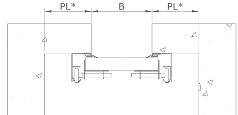
Pealtvaade
